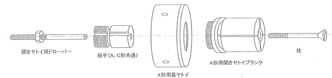
B形開きヤトイ装置
