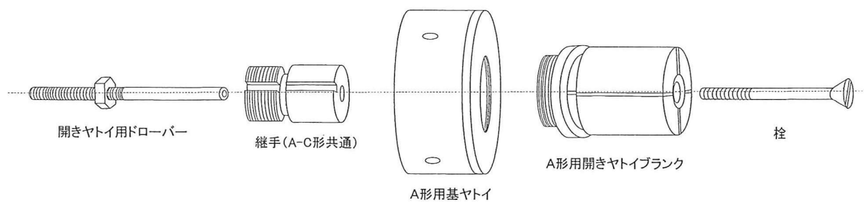
8号 A形開きヤトイ装置
